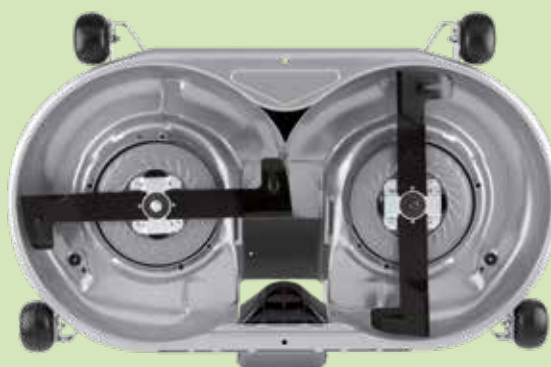
Asynkroniserte kniver
